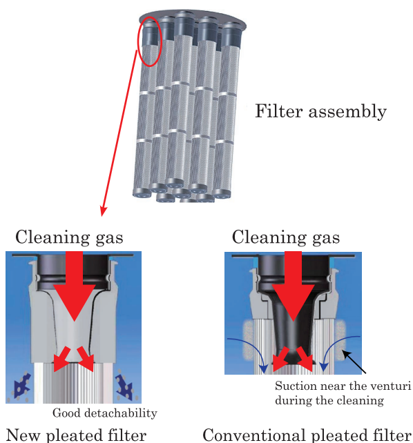
図9 ベンチュリ内蔵型フィルタと従来型の違い
