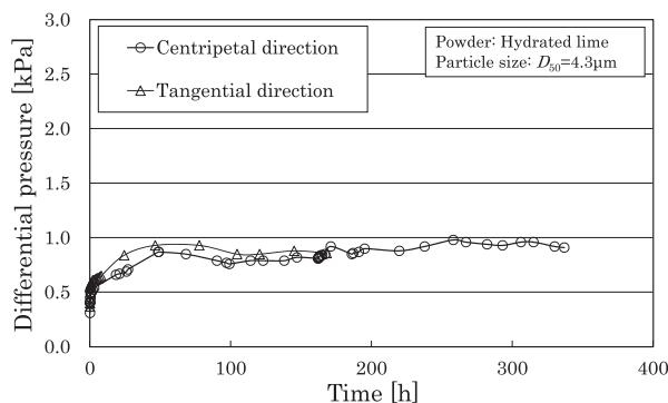
図8 インレット方向とフィルタ差圧
