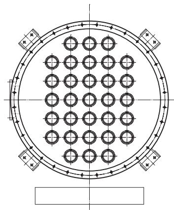
図6 フィルタ配列例 Fig. 6 An example of filter arrangement.
