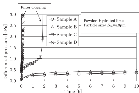
図4 実証試験結果例 Fig. 4 An example of demonstration test.
